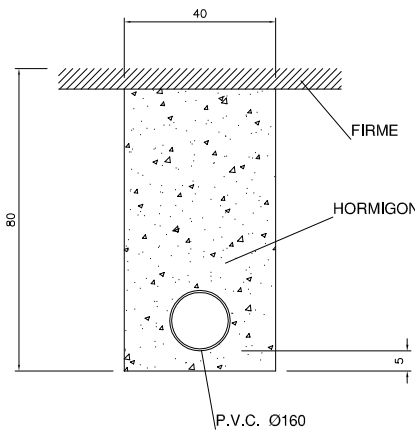
ZANJA CALZADA
