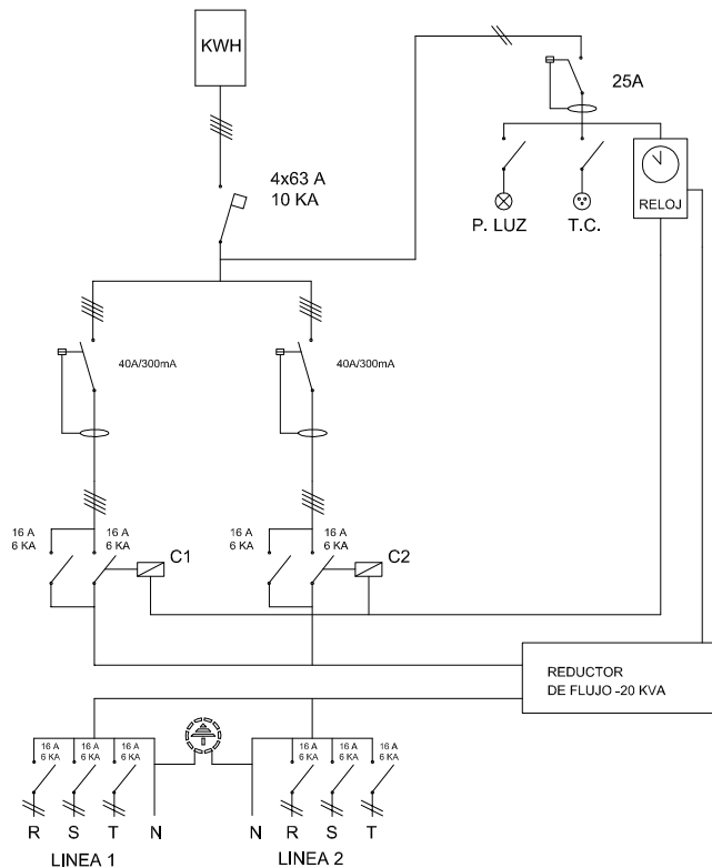
ESQUEMA ELÉCTRICO
