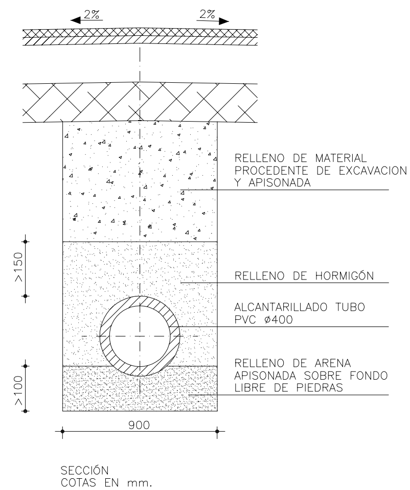
ZANJA CANALIZACIÓN SANEAMIENTO
