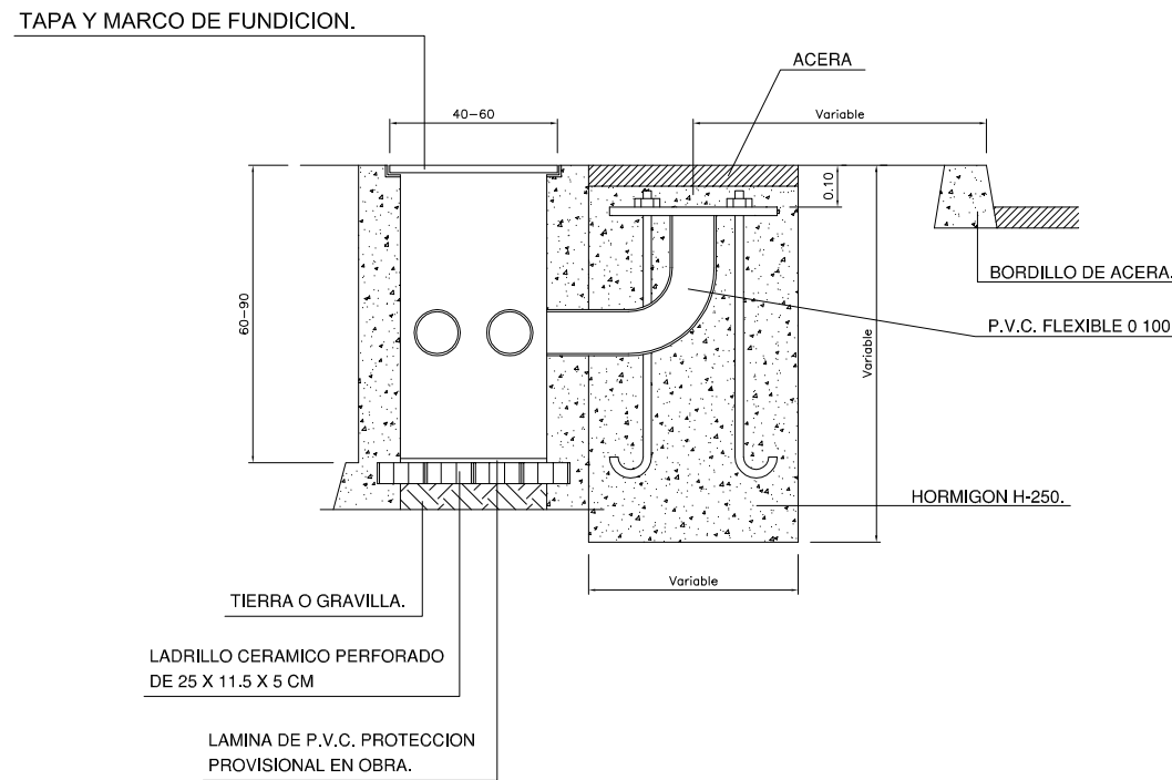
DETALLE CIMENTACIÓN COLUMNA CON ARQUETAS
