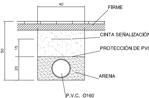
ZANJA ACERAS
