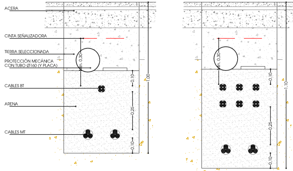
CANALIZACIONES MEDIA Y BAJA TENSION EN ACERAS
